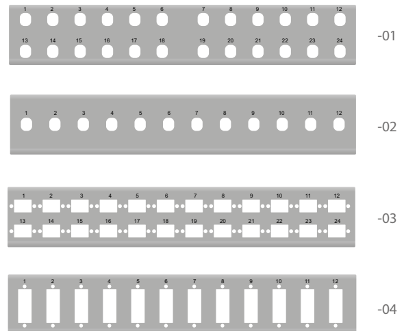
Verteilerplatte
