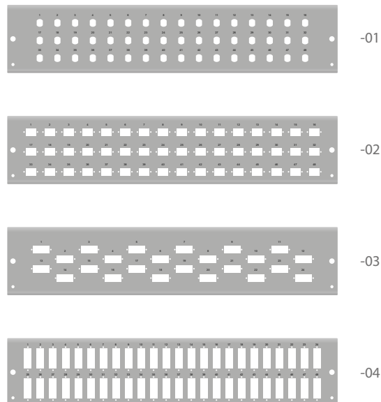
Verteilerplatte
