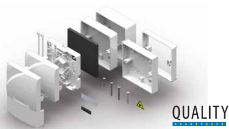
Spleißdose mit optionalem Zubehör
